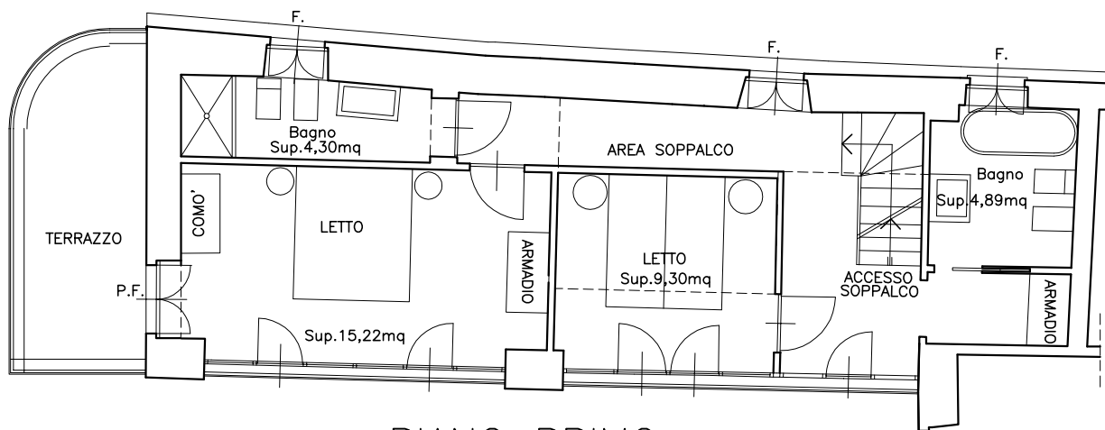
PIANO PRIMO
